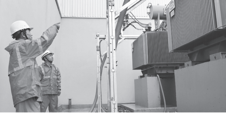
Điện lực Hải Lăng đưa vào vận hành nhiều trạm biến áp công suất lớn để cung ứng điện liên tục, an toàn, hiệu quả - Ảnh: V.M
